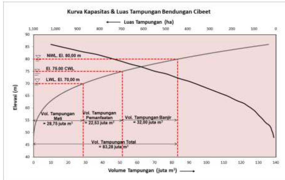
Gambar 4.5. Kurva Kapasitas dan Luas Tampung Bendungan Cibeet
