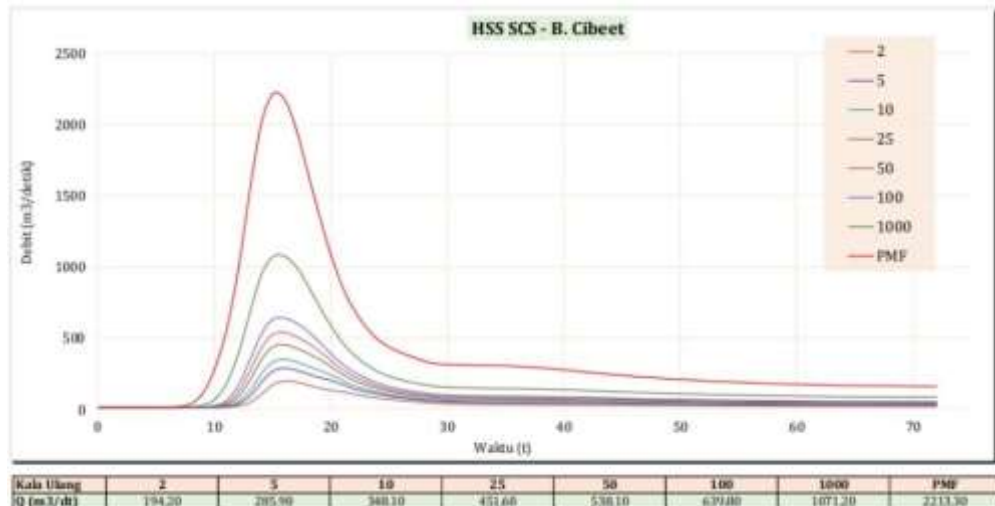
Gambar 4.3. Grafik Banjir Rancangan
