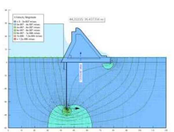
Gambar 4.10. Rembesan Pada Muka Air Banjir
