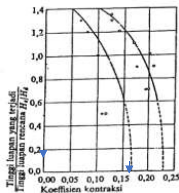
Gambar 4.6. Grafik Hubungan K_a dan h/H_d
