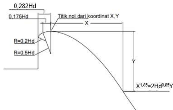
Gambar 4.8. Persamaan Perencanaan Mercu Spillway
